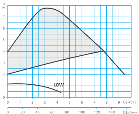
Пропорциональное давление
