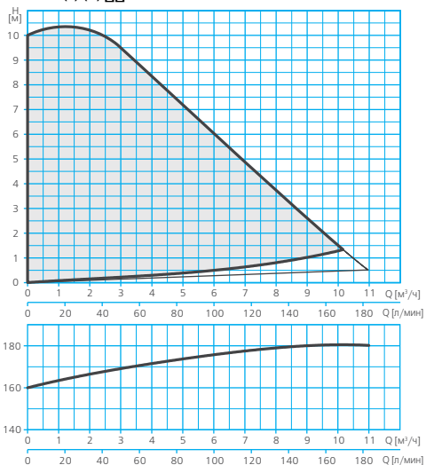
RE2-S(F) (X) _-100
