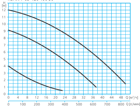
RSAN-F 65-120 400 50
