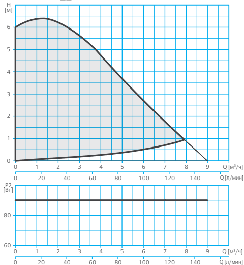
RE2-S(F) (X) _-60
