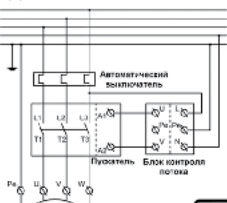
Подключение насоса к сети 3-400 В
