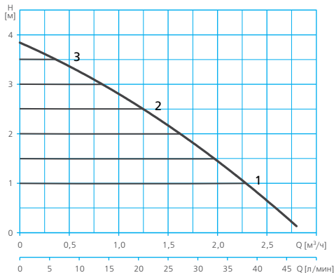
Постоянное давление
