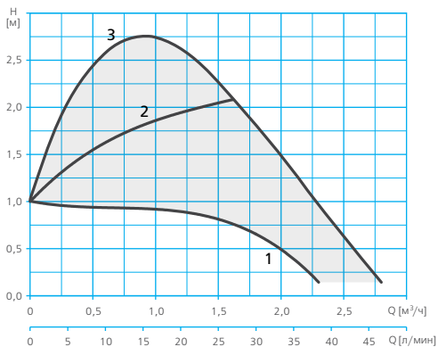
Пропорциональное давление
