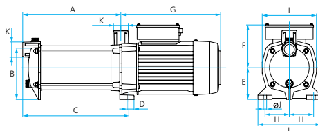
PRISMA25 6
