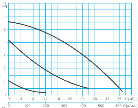
RSAN-F 65-70 400 50
