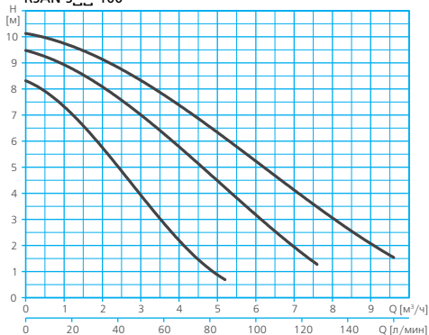
RSAN-S...-100
