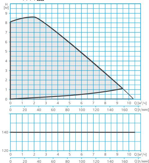
RE2-S(F) (X) _-80
